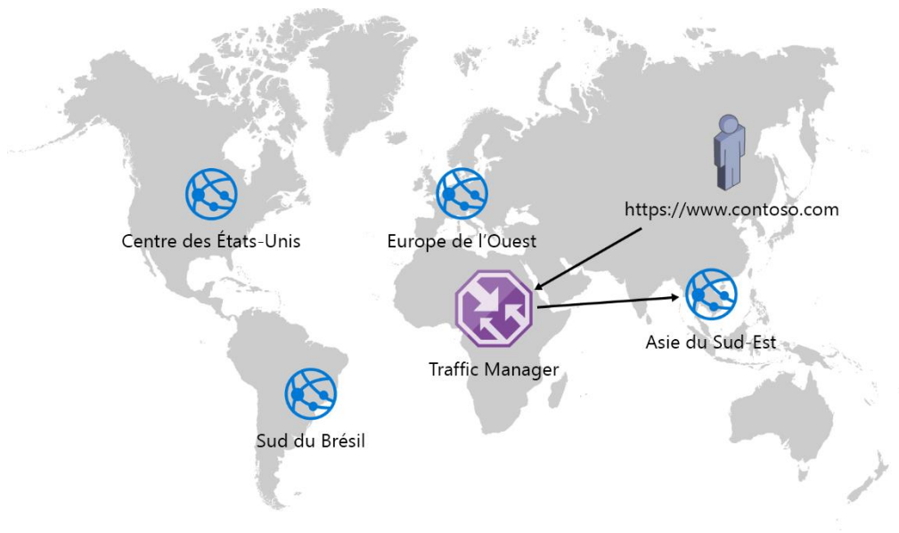
Figure 2-2 : Azure Traffic Manager redirige le trafic vers le point de terminaison géographique le plus performant
