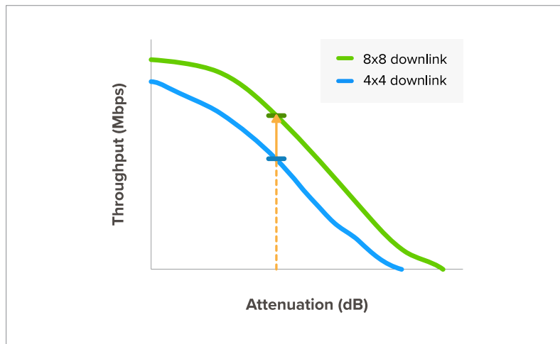
Schéma 8. Amélioration de la fiabilité RF pour un client 3x3 avec une architecture 8x8 par rapport à une architecture 4x4
