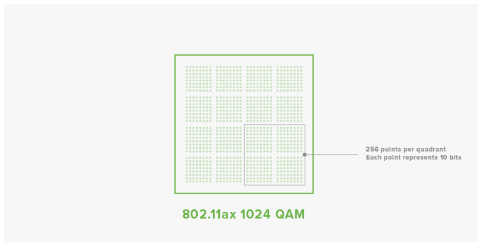
Schéma 9. Modulation 1024-QAM avec le Wi-Fi 6 (10 bits par symbole)
